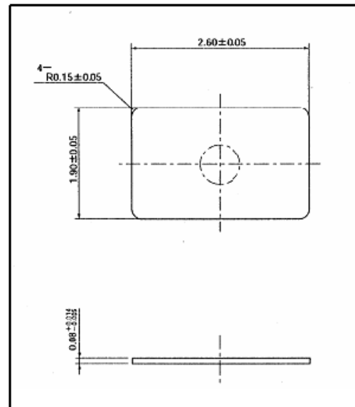
【2.6×1.9 DIMENSION】
