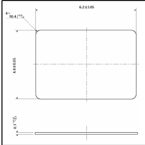
【7×5 DIMENSION】
