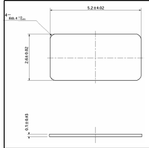
【6×3.5 DIMENSION】
