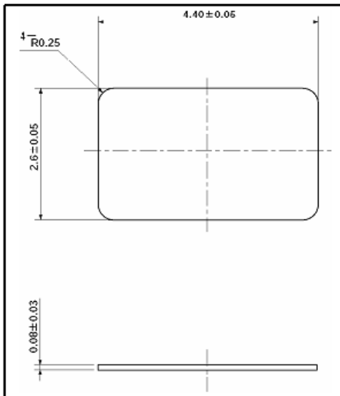
【5×3.2 DIMENSION】
